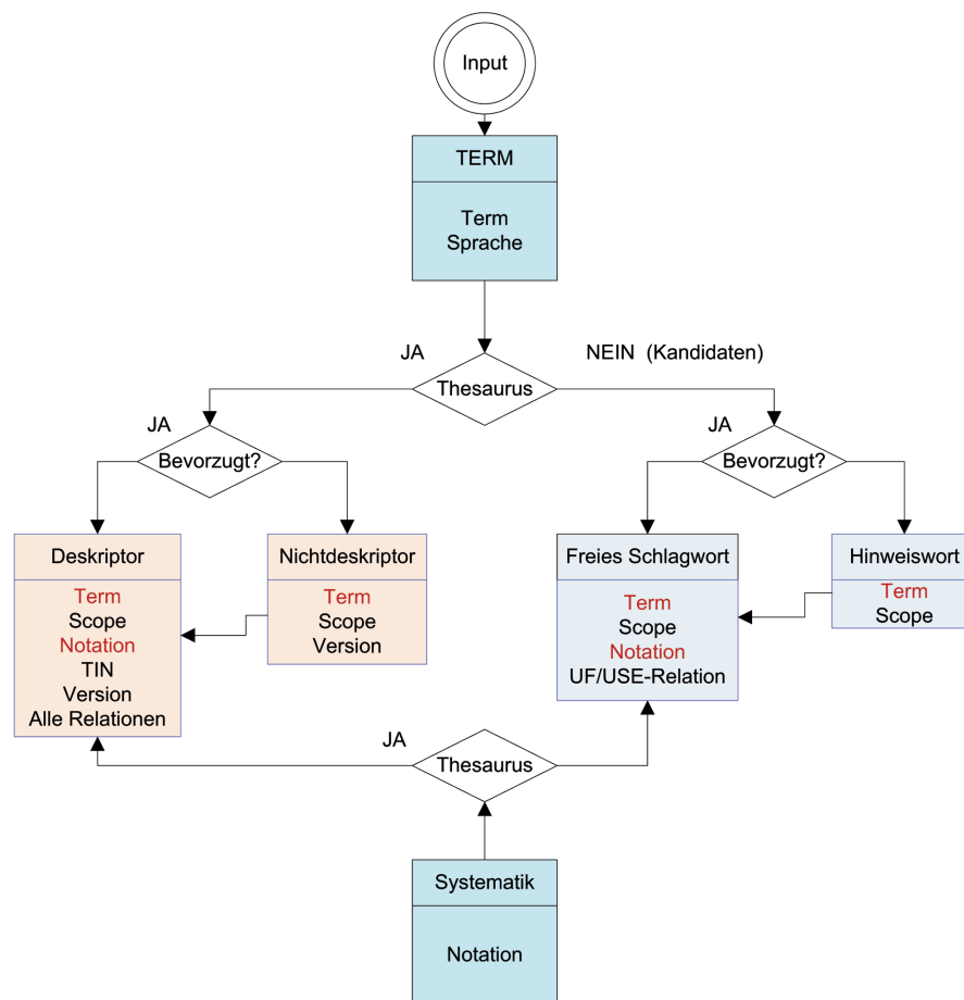
Abbildung 2: Thesaurusmodell.
